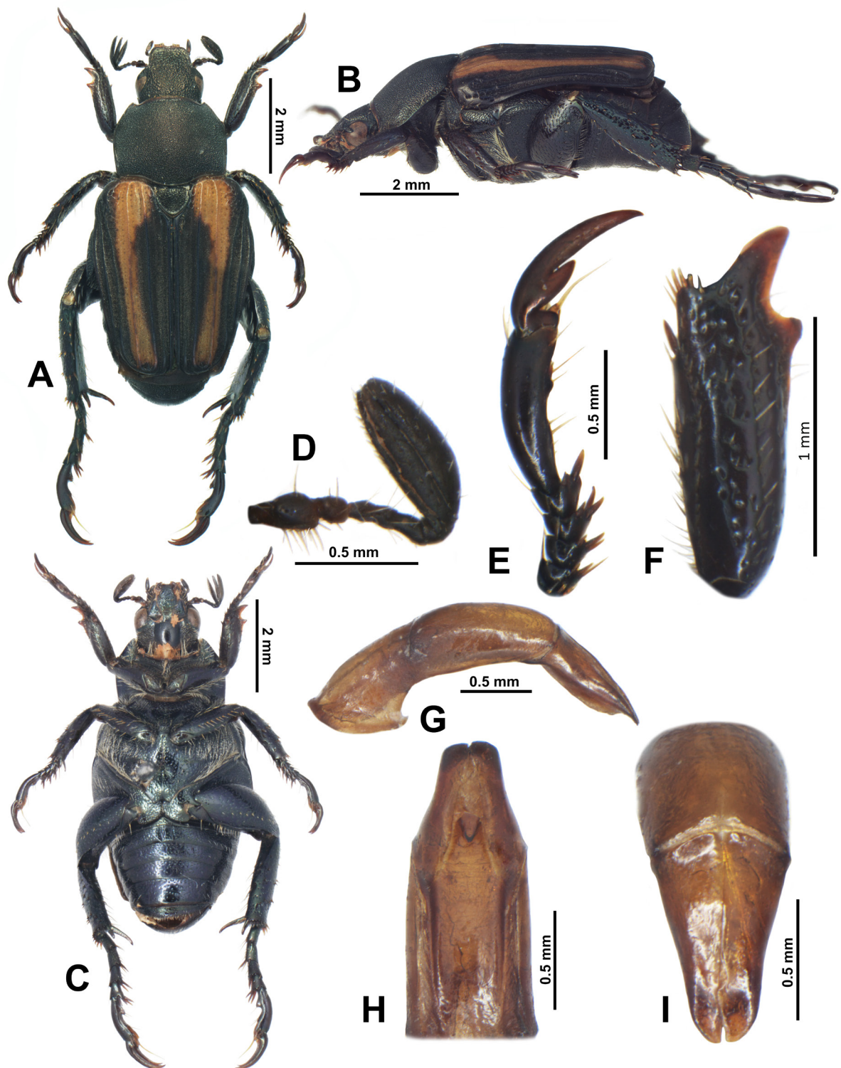
Fig. 9. Strigoderma (Costatergus) juliani Andalco-Cid & Ramírez-Ponce subgen. et sp. nov., holotype, ♂ (UNSM). A. Dorsal habitus. B. Ventral habitus. C. Lateral habitus. D. Antenna. E. Protarsus. F. Protibia. G–I. Genitalia. G. Lateral view. H. Ventral view. I. Frontal view.
